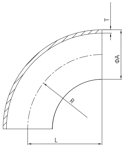
ISO1127 90° 弯头
