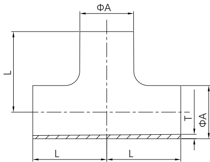
ISO1127 等径三通
