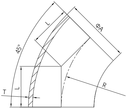
ISO1127 45° 弯头
