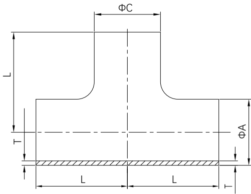
ISO1127 变径三通
