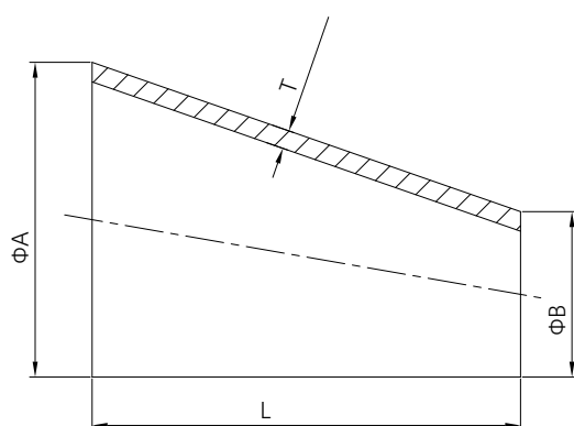
ISO1127 偏心变径
