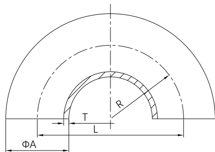
ISO1127 180° 弯头
