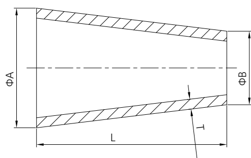
ISO1127 同心变径
