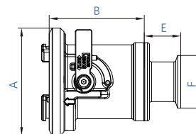
807型 卡箍连接
