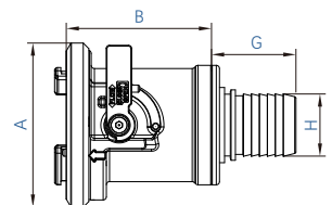
808型 宝塔连接
