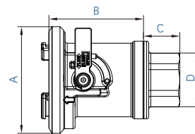
801型 螺纹连接
